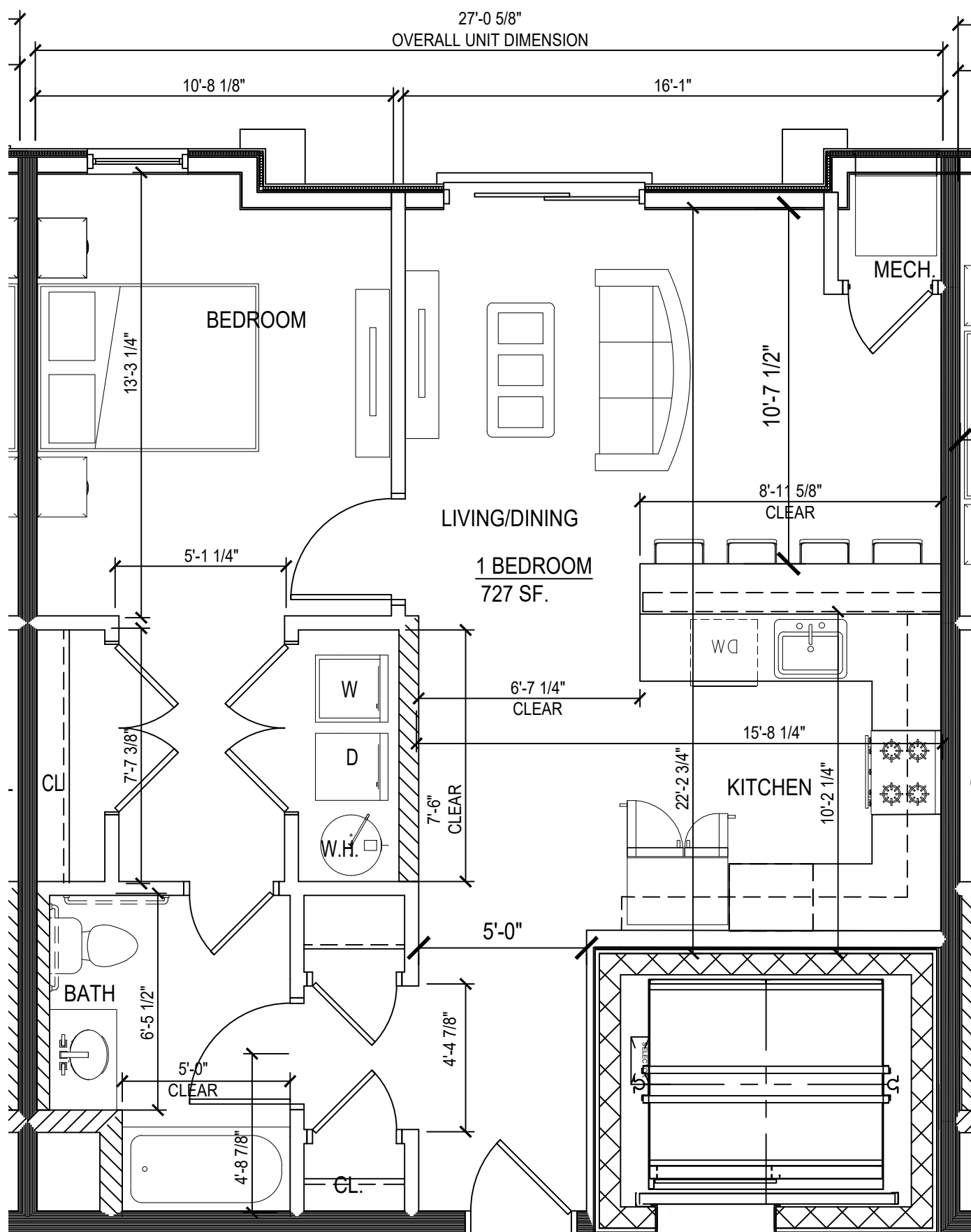
1 UNIT 217 - 317 - 1 BED ROOM - 727 S.F. SCALE: 1/4"=1'-0"
