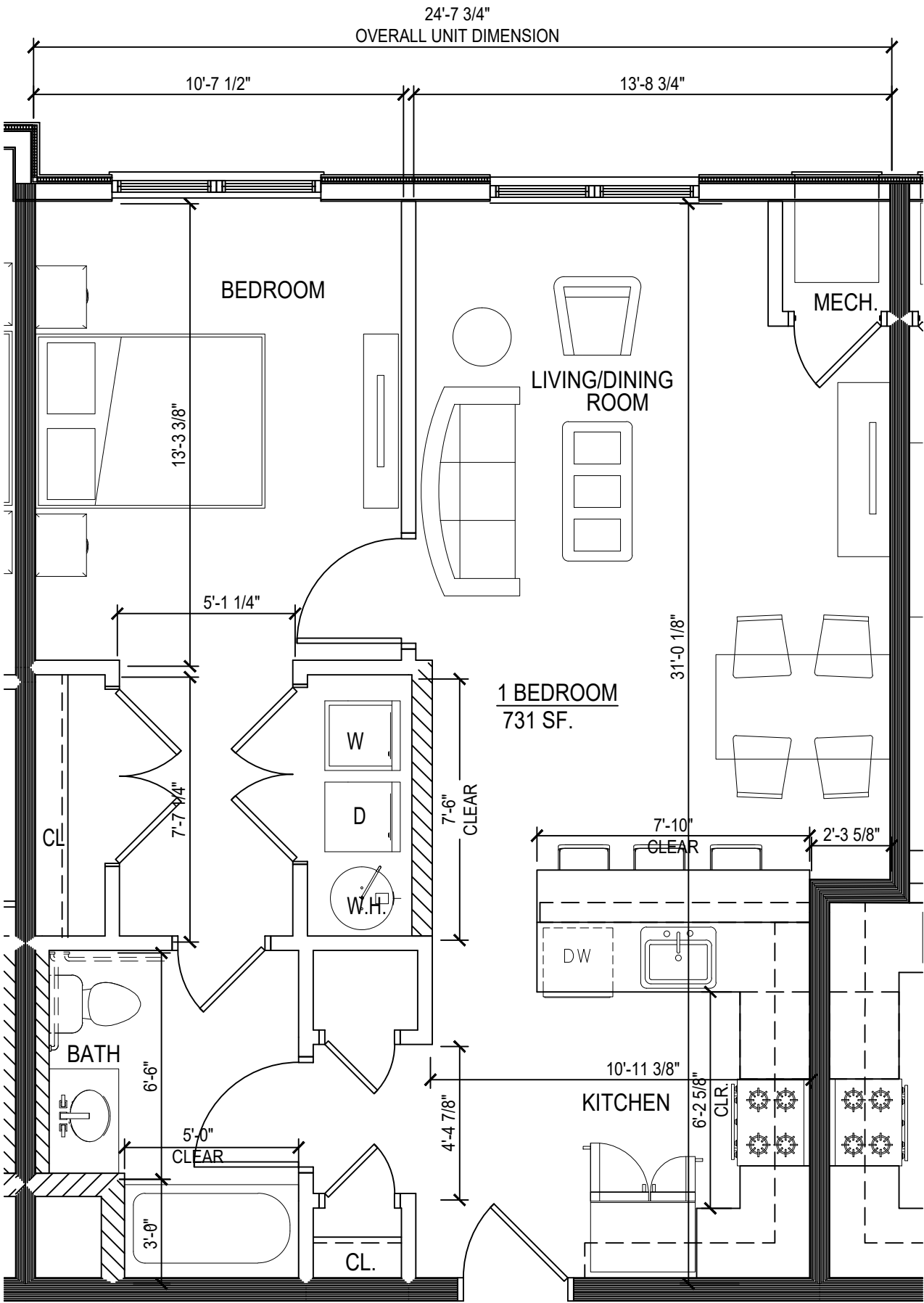
1 UNIT 215 - 315 - 1 BED ROOM - 731 S.F. SCALE: 1/4"=1'-0"
