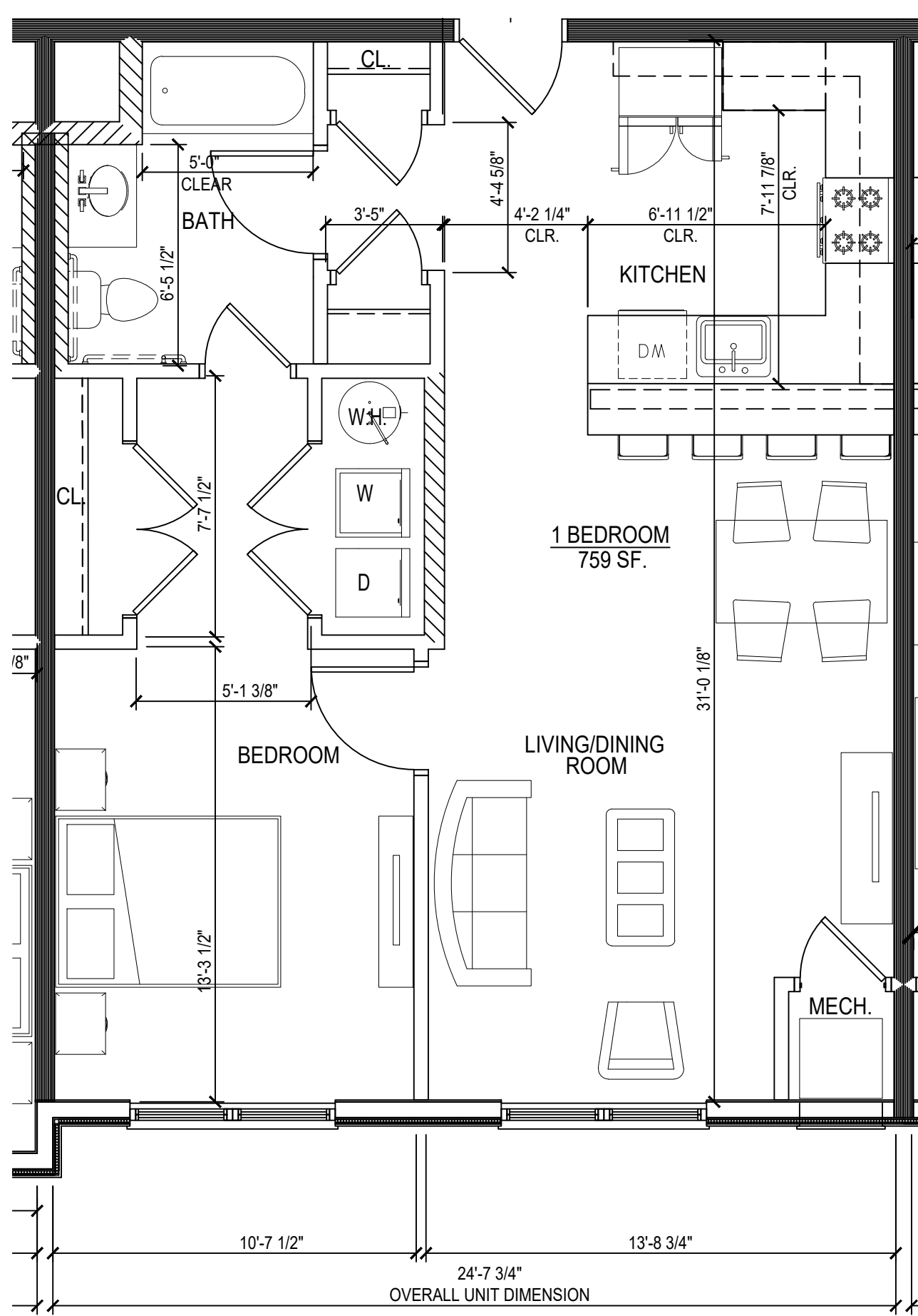
1 UNIT 210 - 310 - 1 BED ROOM - 759 S.F. SCALE: 1/4"=1'-0"
