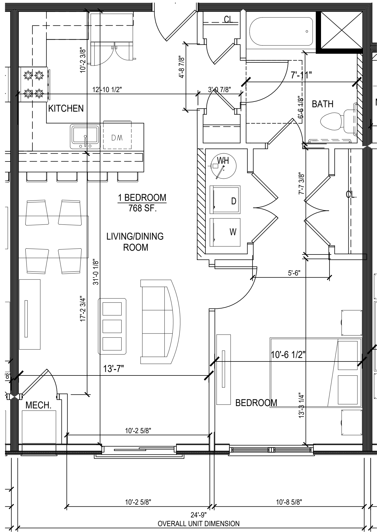
1 UNIT 209, 309 - 1 BED ROOM - 768 S.F. SCALE: 1/4"=1'-0"
