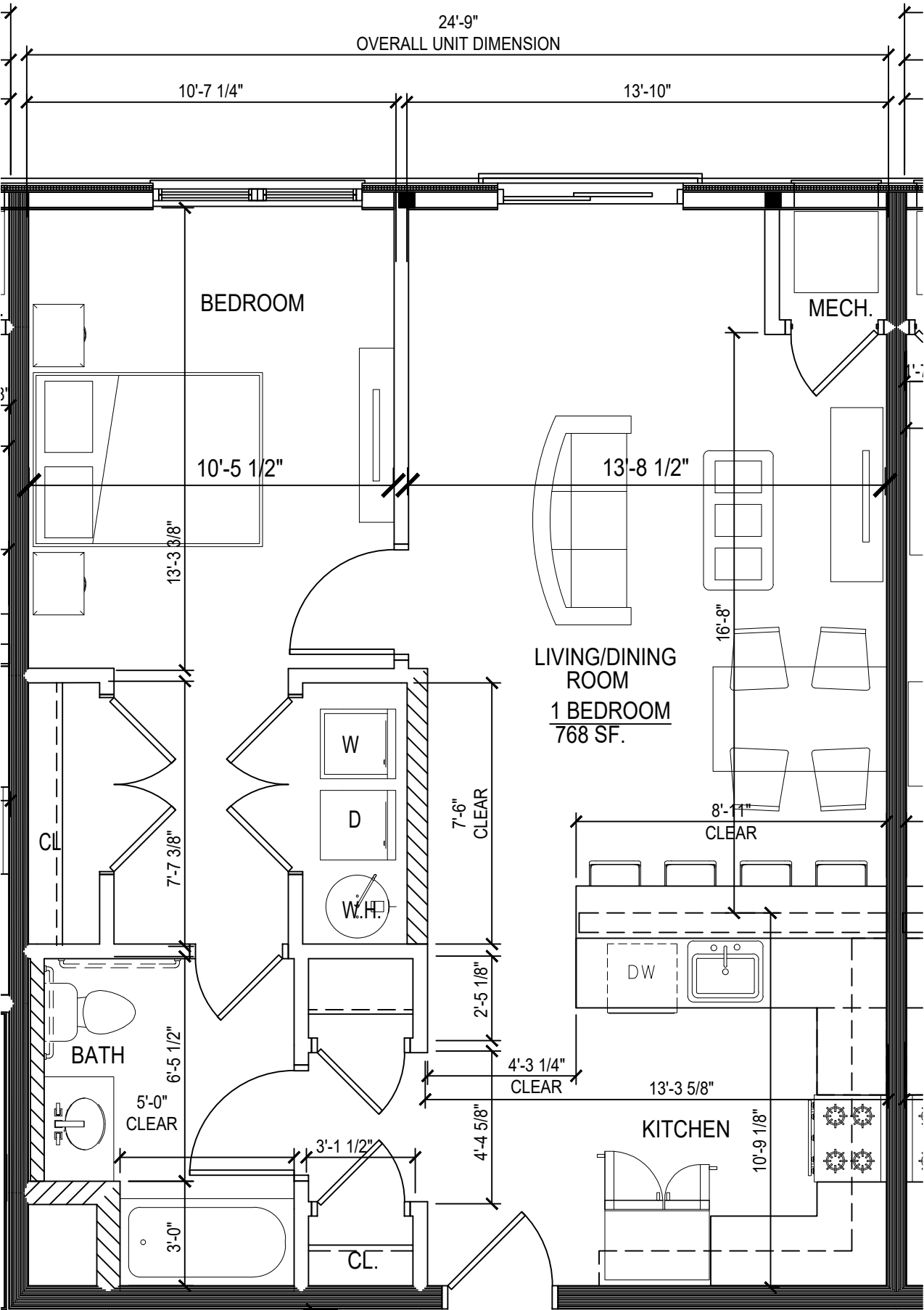
1 UNIT 201, 301 - 1 BEDROOM - 768 S.F. SCALE: 1/4"=1'-0"
