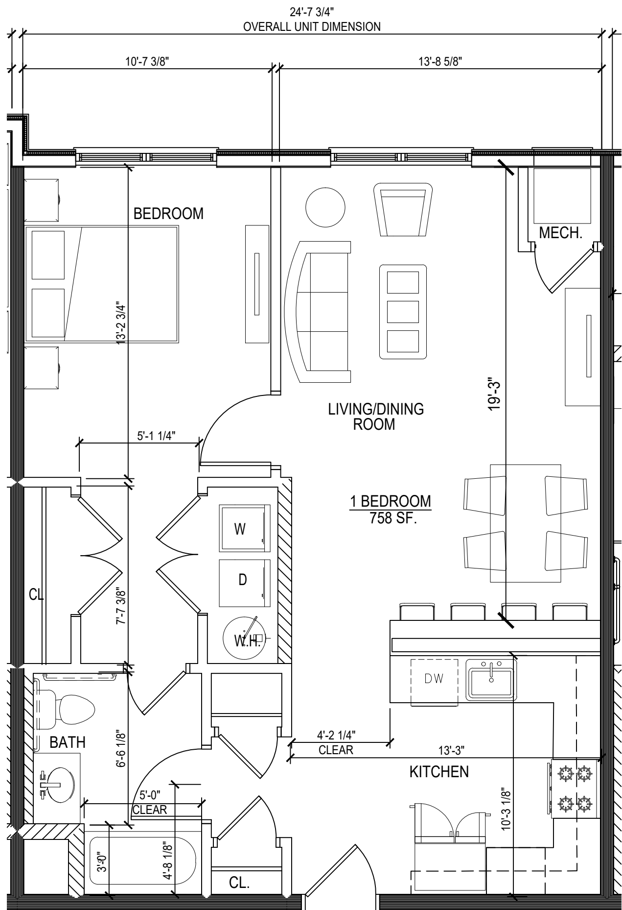
1 UNIT 116 - 1 BED ROOM - 758 S.F. SCALE: 1/4"=1'-0"
