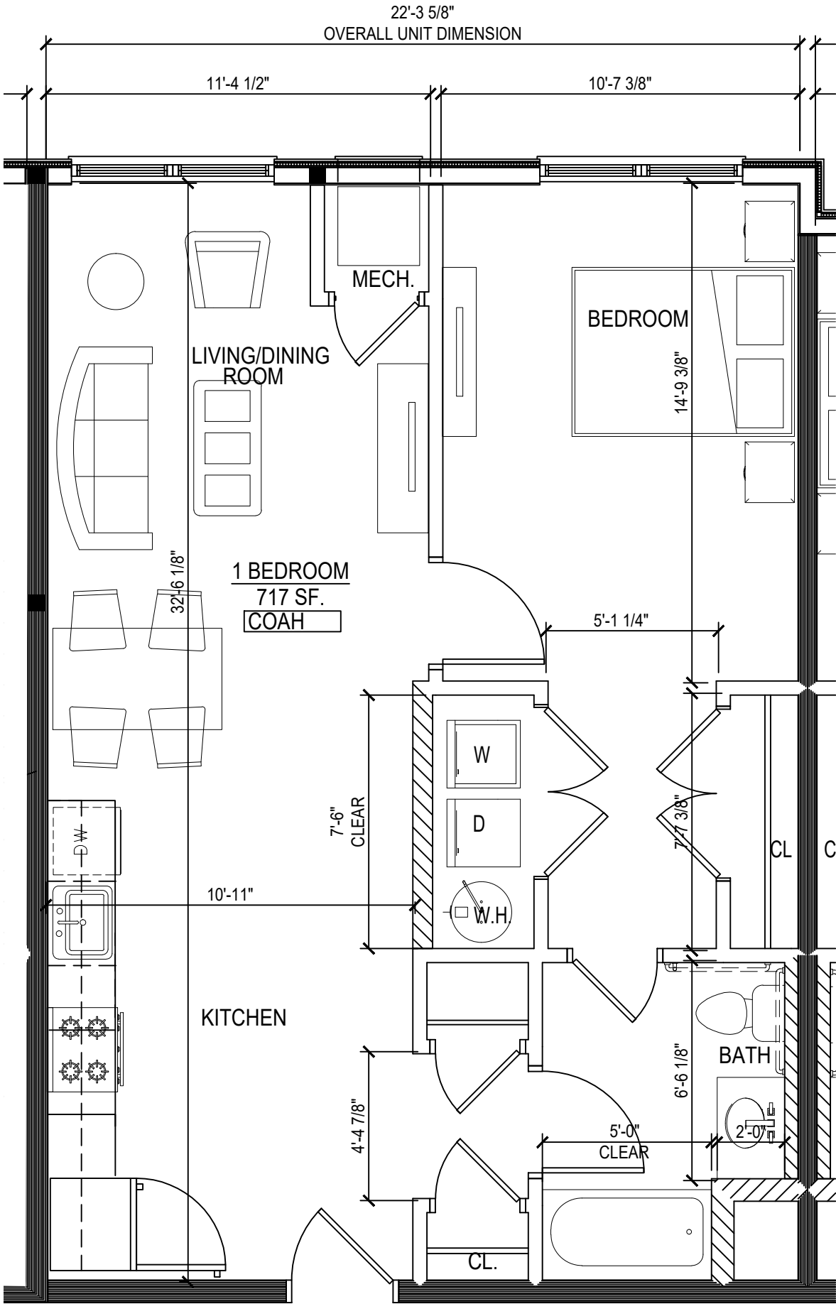
1 UNIT 115 - 1 BED ROOM - 717 S.F. SCALE: 1/4"=1'-0"
