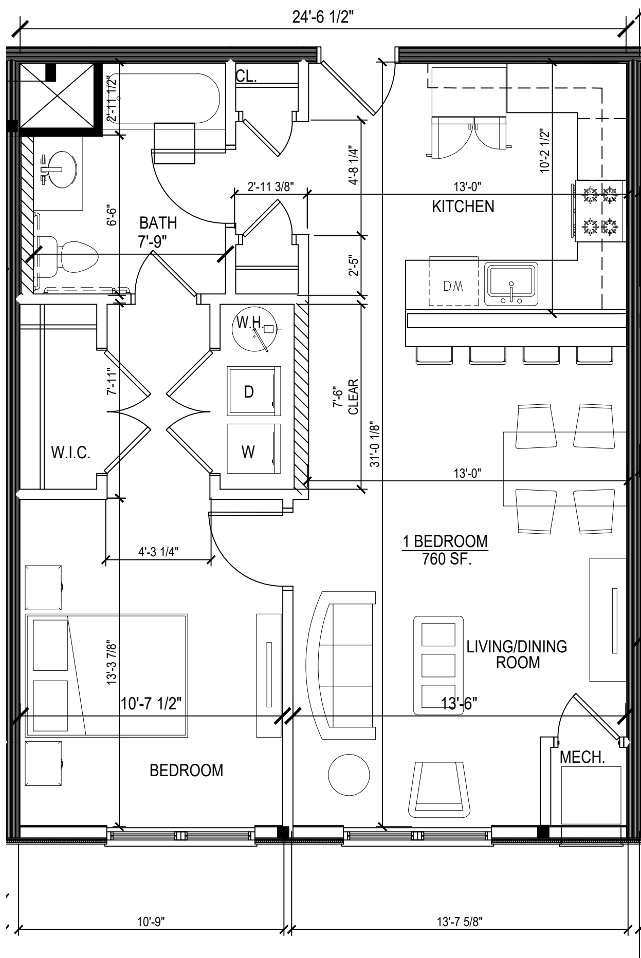
1 UNIT 108 - 1 BDRM - 760 S.F. SCALE: 1/4"=1'-0"
