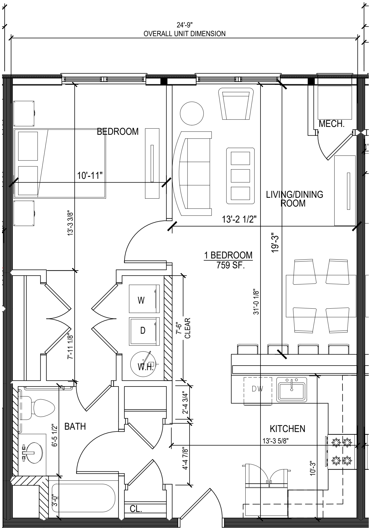
1 UNIT 101 - 1 BDRM - 759 S.F. SCALE: 1/4"=1'-0"
